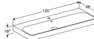
WASTAFEL 120 CM SQUARE Met kraangat, met overloop Zonder kraangat, met overloop Zonder kraangat, met overloop, KeraTect® Met twee kraangaten, met overloop Met twee kraangaten, met overloop, KeraTect®
